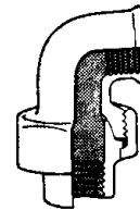
FIG. 096 BOCCHETTONE A GOMITO MASCHIO FEMM. SEDE PIANA DA 1/2" A 3"
