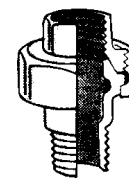
FIG. 341 BOCCHETTONE MASCHIO FEMMINA SEDE CONICA DA 1/4" A 4"
