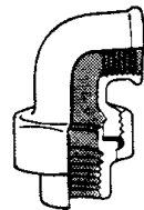
FIG. 095 BOCCHETTONE A GOMITO FEMMINA FEMMINA SEDE PIANA DA 1/2" A 2"
