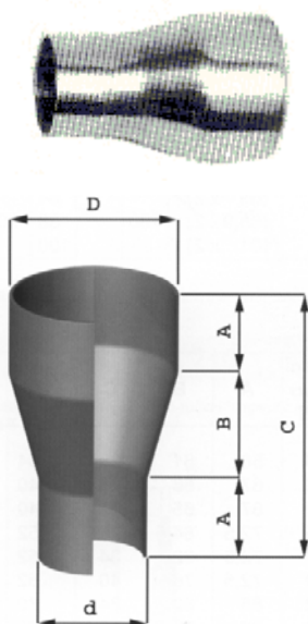
ART. RMM 236 RIDUZIONE CONCENTRICA
