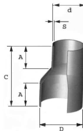
ART. RMM 237 RIDUZIONE ECCENTRICA
