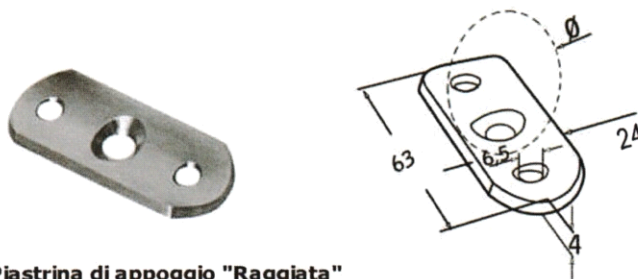
Piastrina di appoggio "Raggiata"
