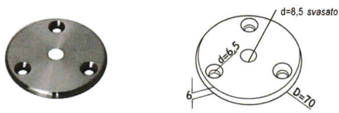
Flangia Ø70 mm
