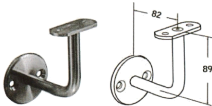
Asta curva fissa "DE"(2 fori)
