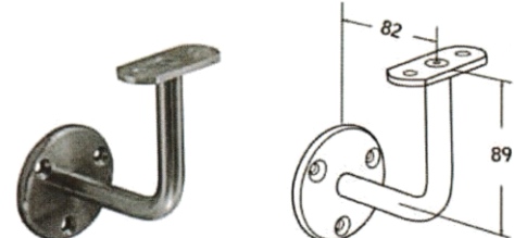
Asta curva fissa "DG"(3 fori)
