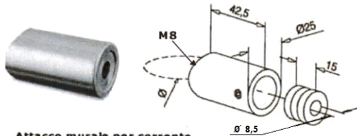
Attacco murale per corrente
