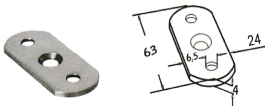
Piastrina di appoggio "Piatta"
