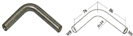
Perno curvo fisso "DE"
