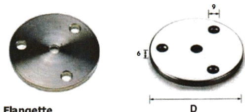
Flangette
