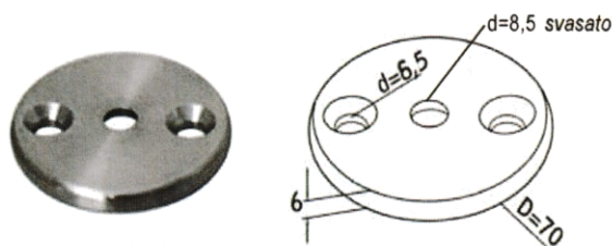
Flangia Ø70 mm
